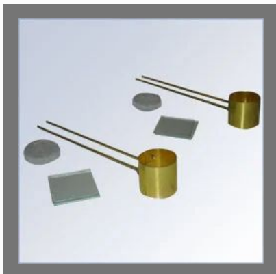
Le-Chatelier Mould
