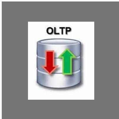
OLTP
