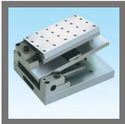
Sine Table
