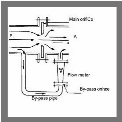
Orifice Flow Meter
