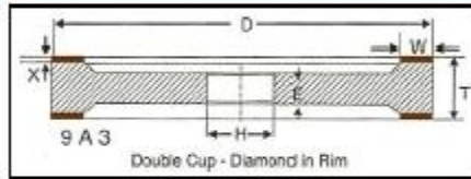
Double Side Cup Type 9A3
