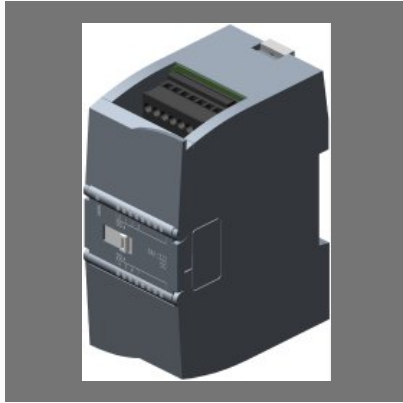
Siemens S7-1200 SM1222 8DO 24V DC
