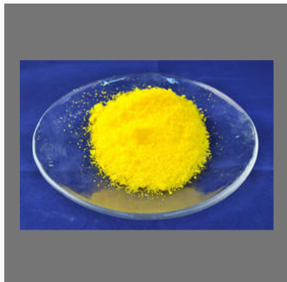
Ammonium Tetra Chloroaurate
