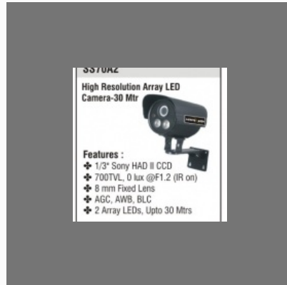
SS70A2 CCD Camera
