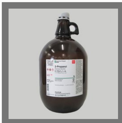
2-Propanol
