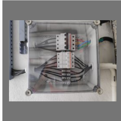
Solar DCDB
