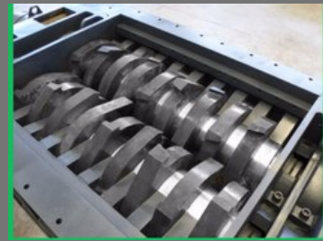
ERS-DSS Dual Shaft Shredder
