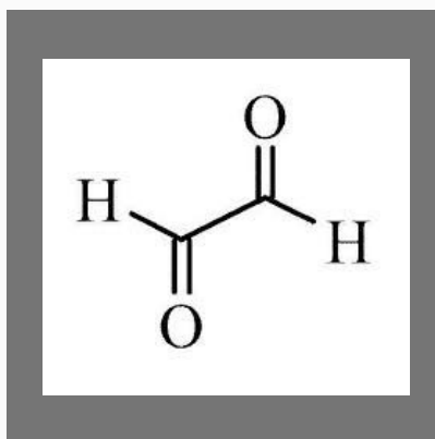
Glyoxal 40%
