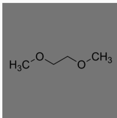
1,2-Dimethoxyethane
