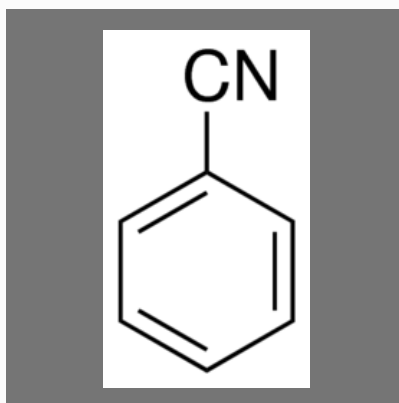
Benzonitrile
