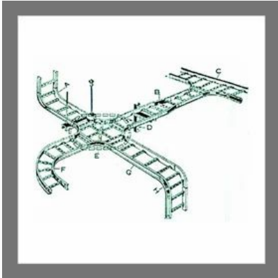
Cable Tray
