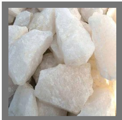
Sodium Feldspar
