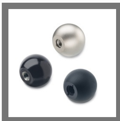
DIN 319 Ball knobs
