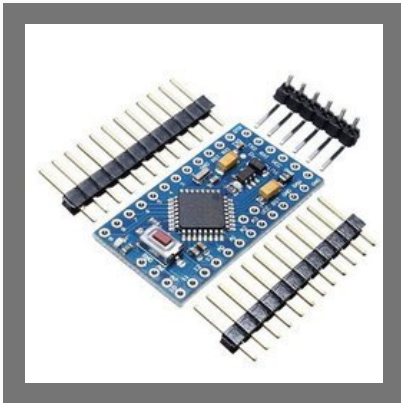
ATMEGA328P Pro Mini 328 Mini ATMEGA328 5V/16MHz for Arduino
