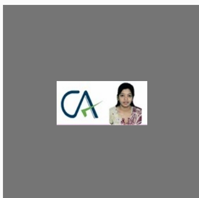
CA Classes
