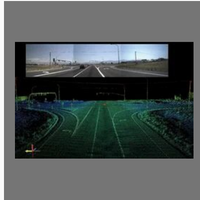
Mobile LIDAR
