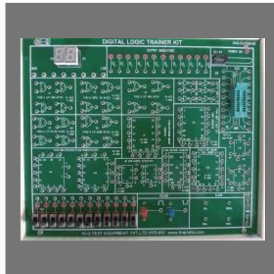
DIGITAL LOGIC TRAINER HiQ UDT604B
