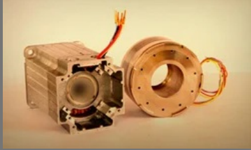
BLDC Motor
