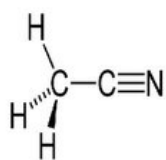
ACETONITRILE
