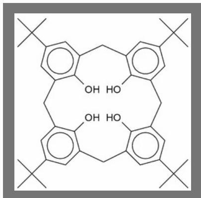
P-terbutyl Calix(4)Arene
