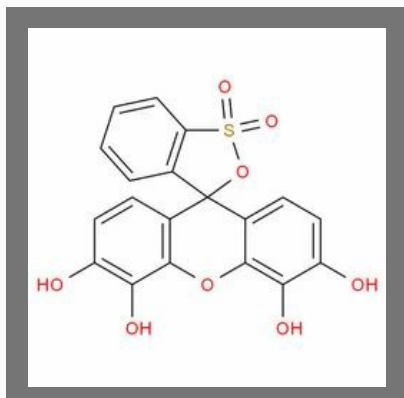
Pyrogallol Red
