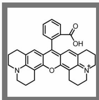
Rhodamine 101
