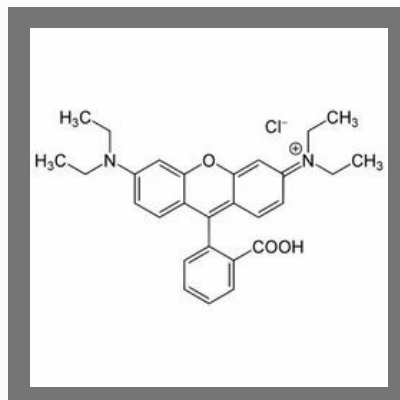
Rhodamine 6G
