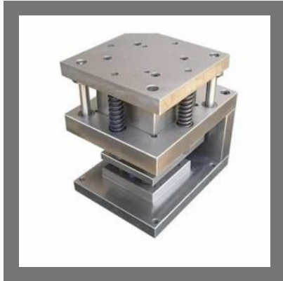
Metal Cutting Die
