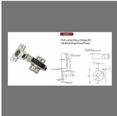
Auto Hinges
