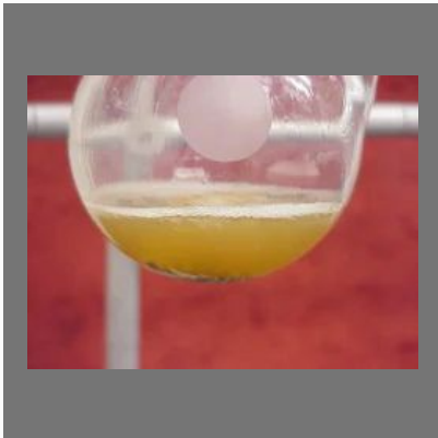
Bromo Benzene Extrapure
