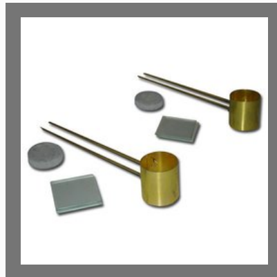
Le Chatelier Mould
