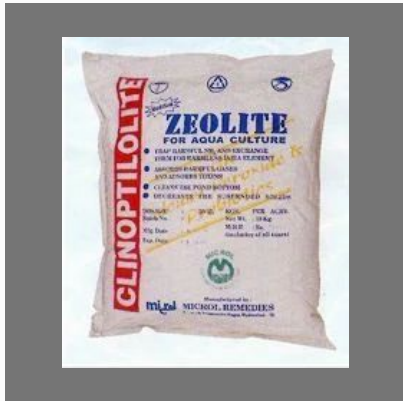
Clinoptilolite
