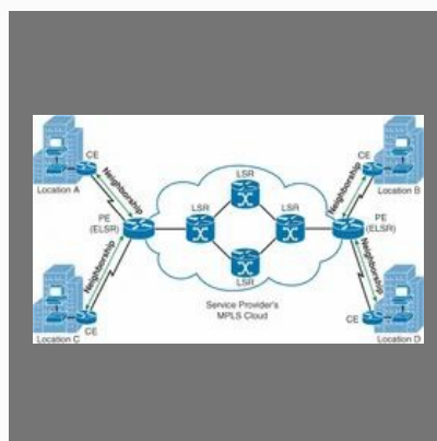
MPLS VPN
