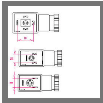
Din Connectors
