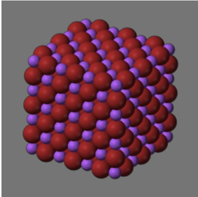
Sodium Bromide
