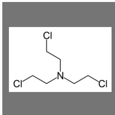
2-Chloroethylamine
