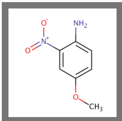
4-Methoxy-2-Nitroaniline
