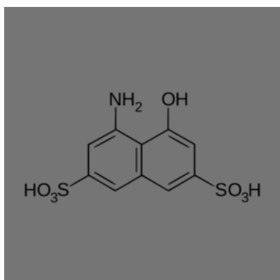
H. Acid
