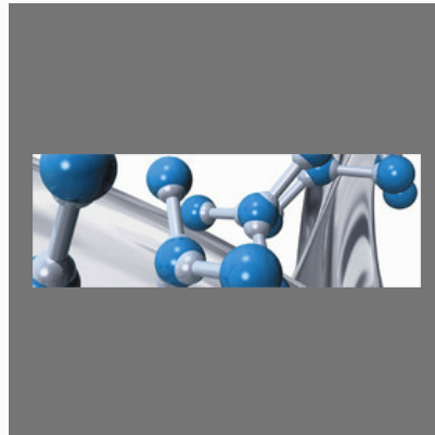
2,3 Dichlorobenzoyl Cyanide
