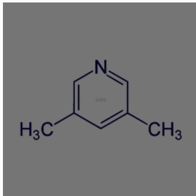
3,5-Lutidine
