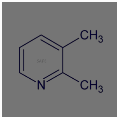
2,3-Lutidine
