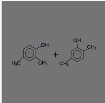
2,4 & 2,5-Xylenol
