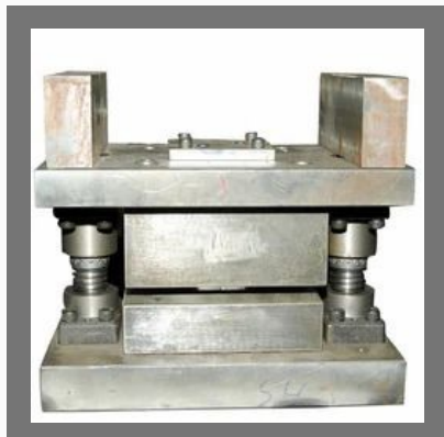
Press Tool
