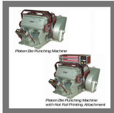
Gurunanak Platen Die Punching Machine
