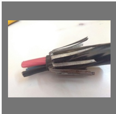
Josnos Cable 1554
