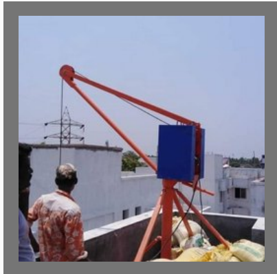
Mini Construction Lift
