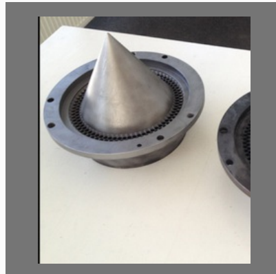
Die Plate
