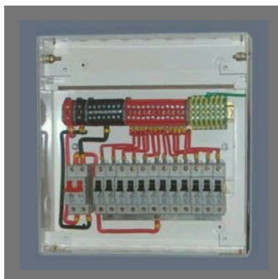
Switch Bord
