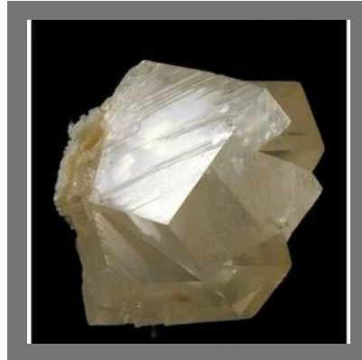
Dolomite Minerals
