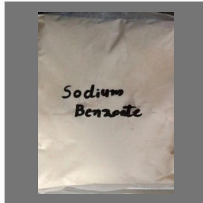
Sodium Benzoate
