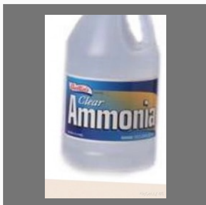
Ammonia
