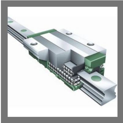
Linear Ball Guide
