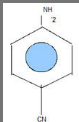
4- Amino Benzonitrile
