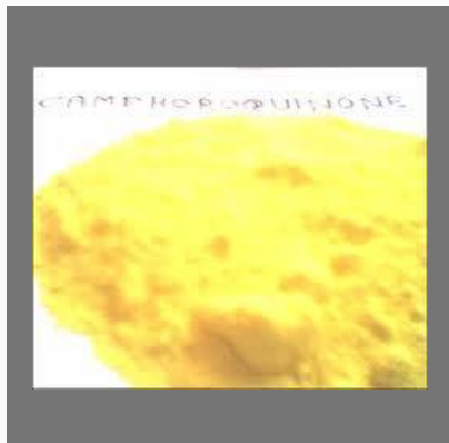
Camphorquinone - C_{10}H_{14}O_2
